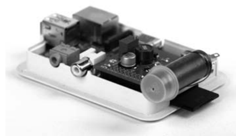
PiGI Geiger-Müller-Zähler
