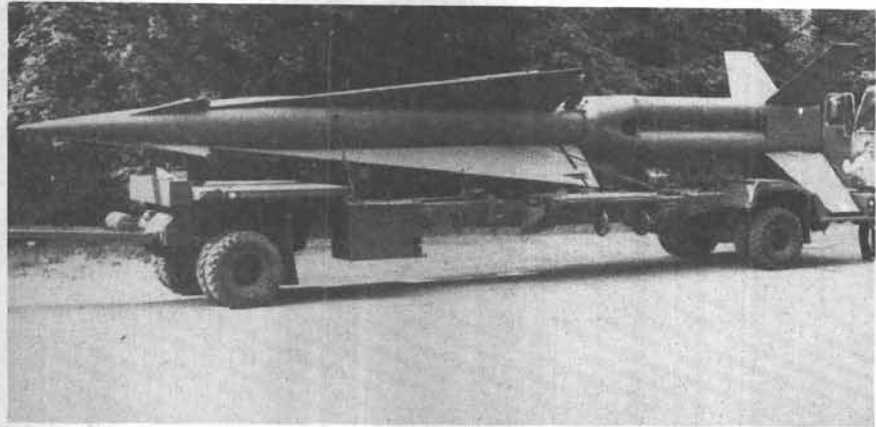
Die Steinbacher Feuerleitstellung liegt an der Ausfallstraße von Giessen kurz vor dem Dorf. Schon von weitem kann man den neuen Radarschirm der kommenden High - Pa - Technologie erblicken, sie steckt unter der riesigen Kuppel.
