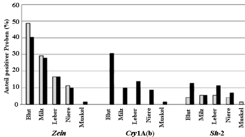
Bild 3. : Anteil positiver Proben (%) des Transgens und von Pflanzengenträgern in fünf Geweben von Tieren der Kontrollen- (●) und Test- (■) Gruppen. Der Prozentsatz positiver Proben für jedes Gewebe wird gerechnet als Anzahl positiver Proben über 72 Beobachtungsreihen (3 PCR-Wiederholungen [Polymerase-Kettenreaktionen] x 3 unabhängige DNS-Isolierungen x 8 Individuen).
