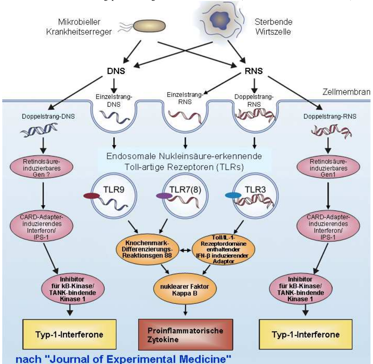
Bild 2: DNS/RNS Erkennungspfade in angeborenen Immunzellen (WAGNER and BAUER 2006)
